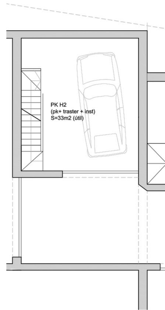
GARATGE (1/100)
