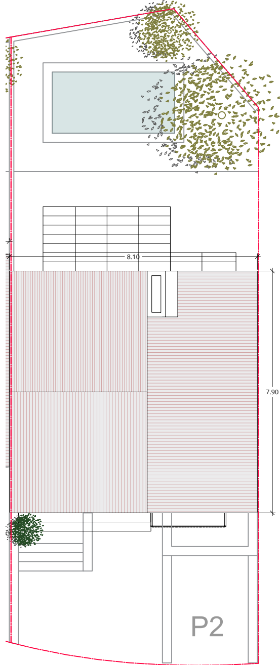
Planta coberta P2
