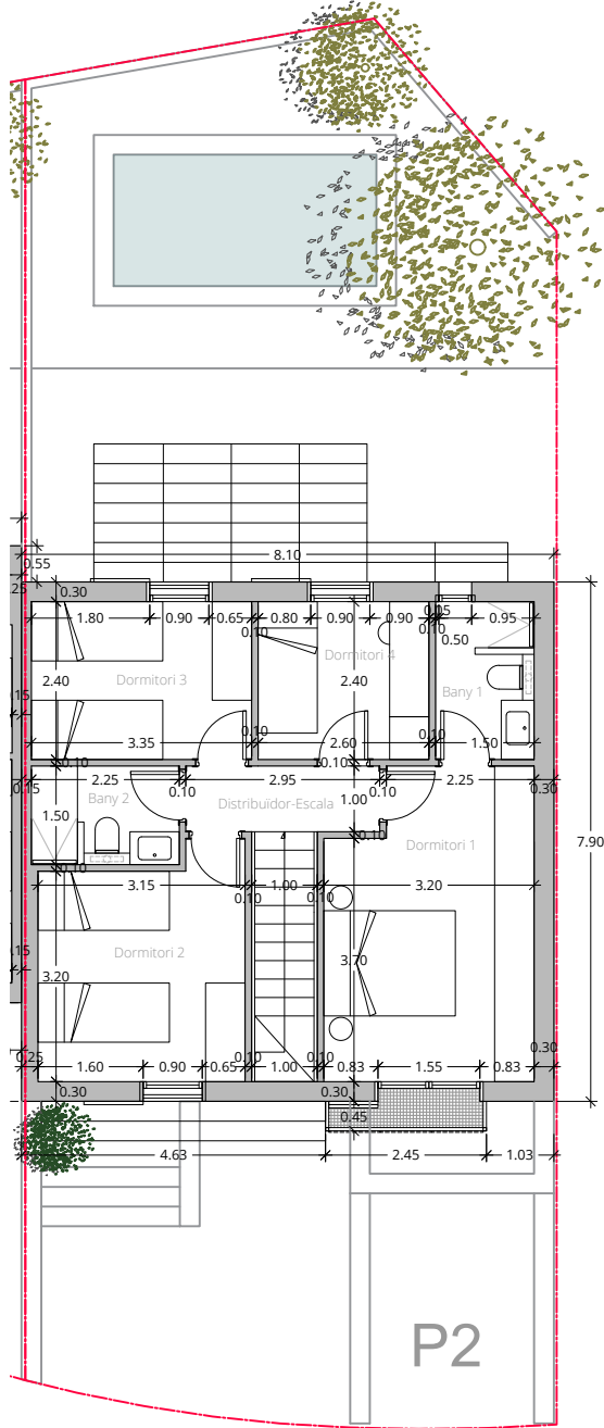
Planta primera P2
