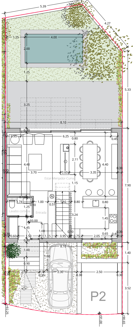
Planta baixa P2
